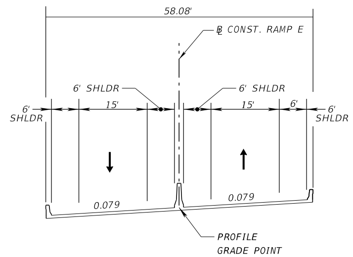
TYPICAL SECTION NO. 23 RAMP E STA. 521+29 TO STA. 523+78
