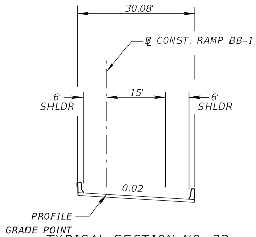
TYPICAL SECTION NO. 22 RAMP B STA. 219+36 TO STA 233+63 RAMP BB-1 STA. 1682+49 TO STA. 1685+53
