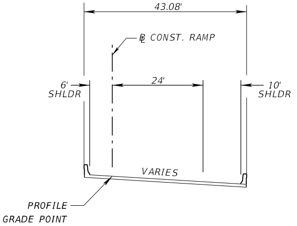
TYPICAL SECTION NO. 21 RAMP C STA. 310+72 TO STA. 321+51 RAMP BB-1 STA. 1664+78 TO STA. 1665+75 RAMP CC STA. 1667.56 TO STA. 1669+31
