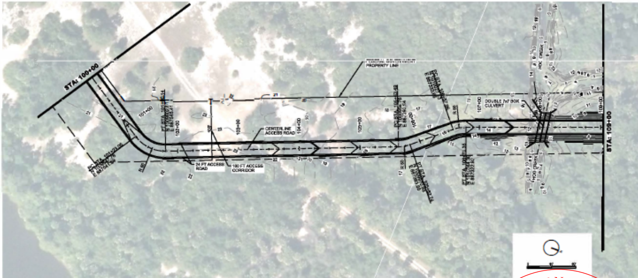
ACCESS ROAD PLAN STA. 100+00 TO STA. 109+00
